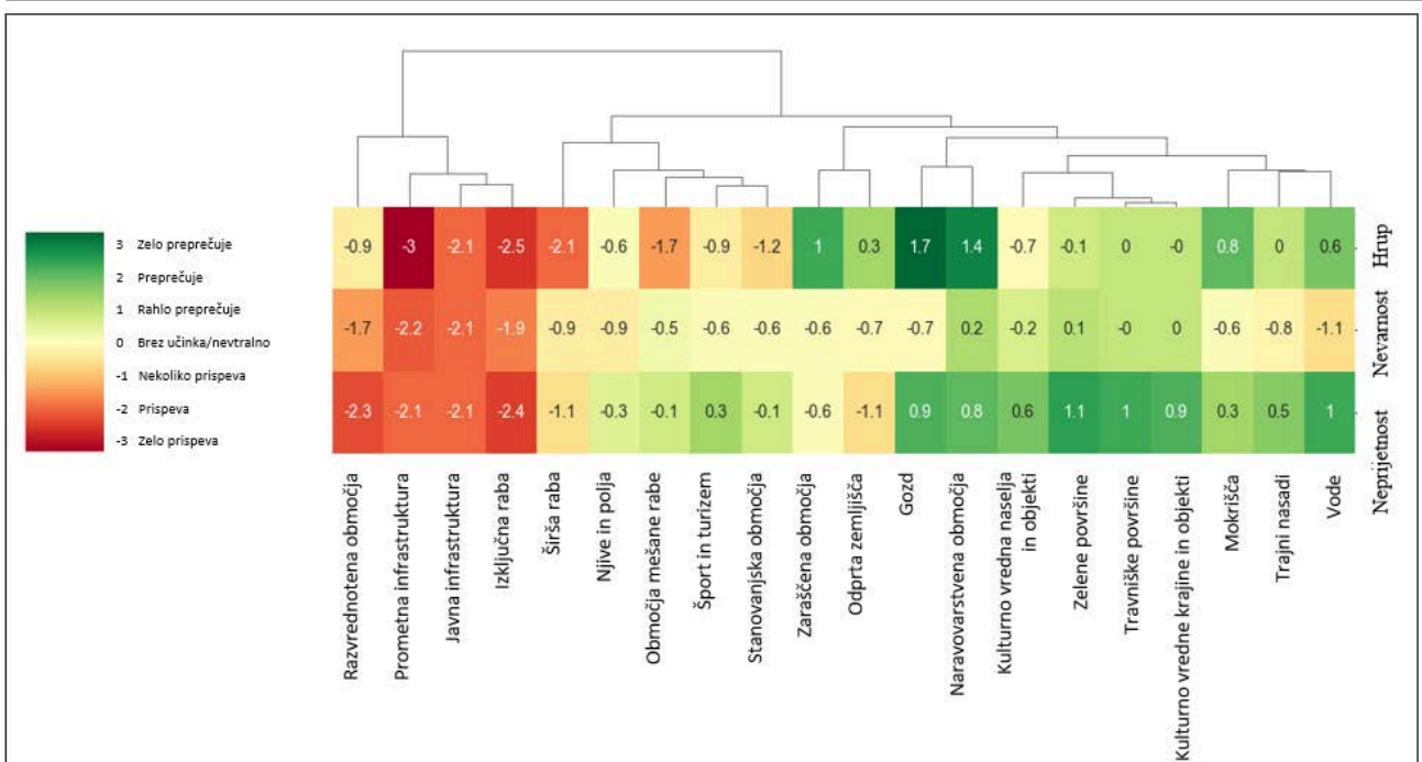
Slika 3: Metoda hierarhičnega razvrščanja v skupine s toplotnim prikazom in dendrogramom, ki ponazarja združevanje tem v skupine za vsako nevršečnost. V vsaki celici je navedena združena povprečna vrednost ocen strokovnjakov, utežena s stopnjo njihovega zaupanja in obarvana z ustreznim odtinkom na barvni lestvici (vir: V. Žlender and S. Gemin)
