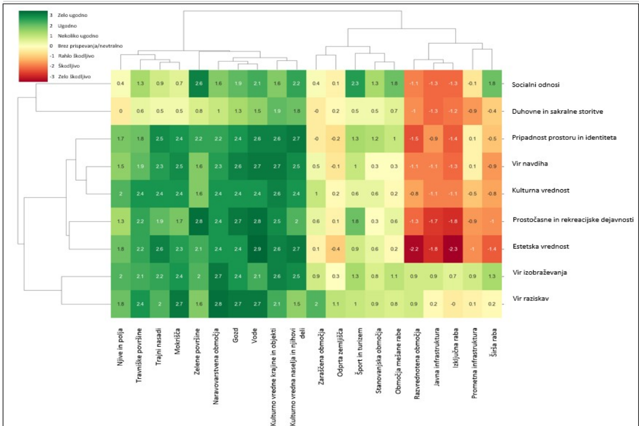
Slika 2: Metoda hierarhičnega razvrščanja v skupine s toplotnim prikazom in dendrogramom, ki ponazarja stolpce združevanja tem in vrstice združevanja KES v skupine. V vsaki celici je navedena skupna povprečna vrednost ocen strokovnjakov, utežena s stopnjo njihovega samozaupanja v odgovor in obarvana z ustreznim odtinkom na barvni lestvici (ilustracija: Vita Žlender in Stefano Gemin)
